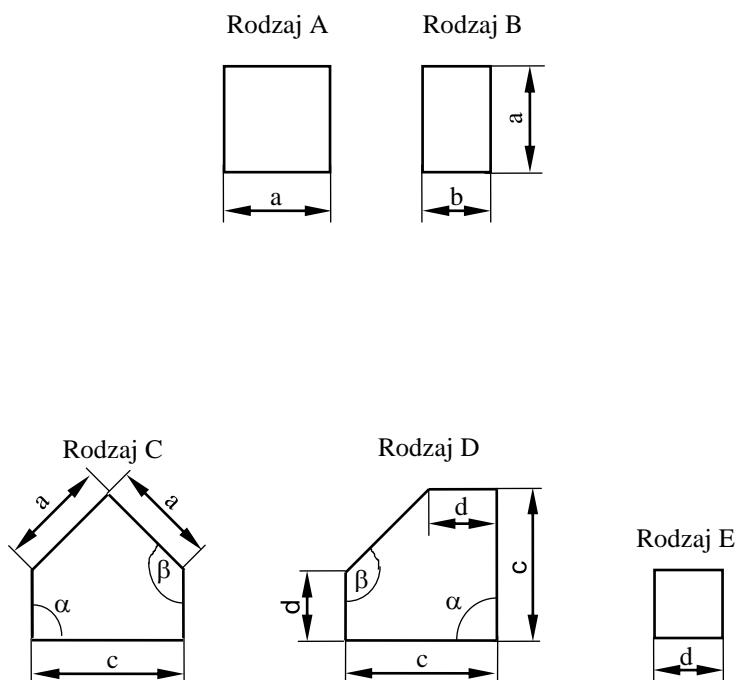
Rysunek 1. Rodzaje płyt chodnikowych betonowych
