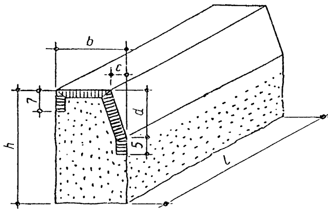
Rys.2. Krawężnik uliczny odmiany UP, rodzaju B
